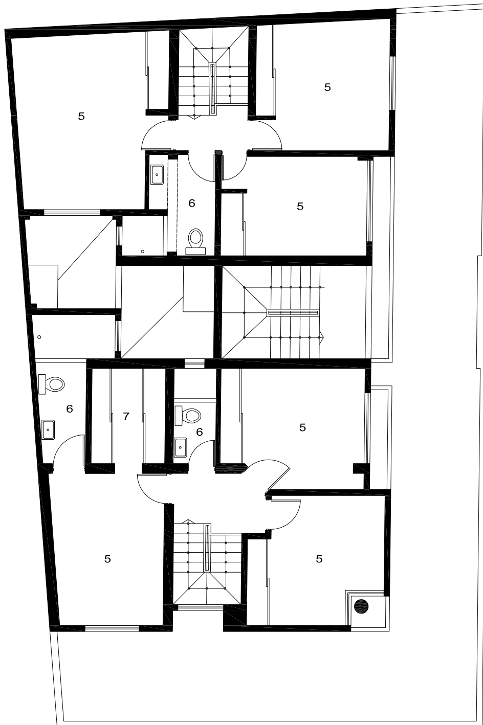
CUARTO PISO
